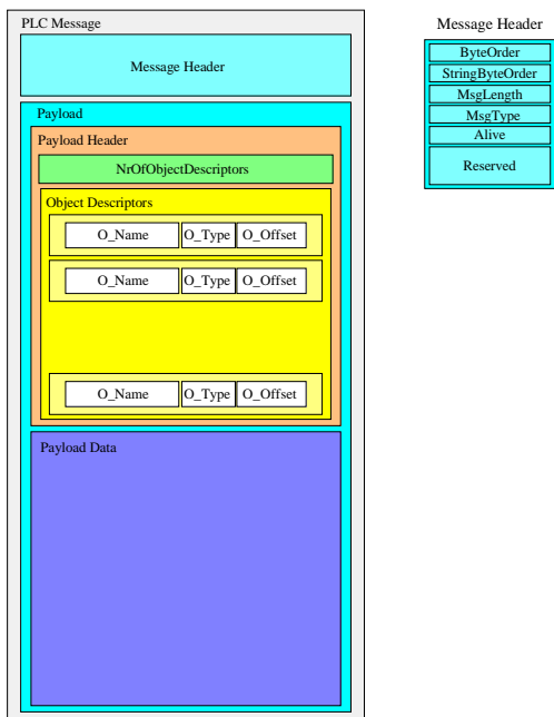
Fig. 4: PLC message format
